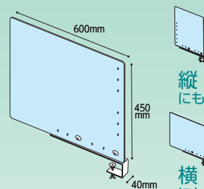
クランプ取付けで、しっかりガード 最大クランプ取付け幅約47mm
